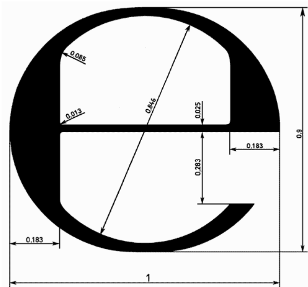
TVAR ZNAČKY „e“
