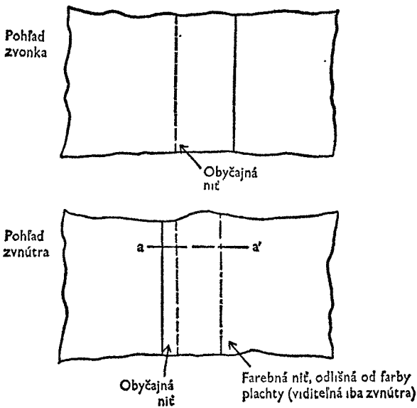
Náčrtok č. 2 Rez vozovou plachtou
