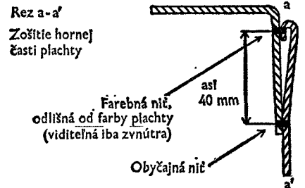
Náčrtok č. 4 Rez vozovou plachtou
