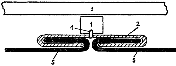
Náčrtok č. 1 Horizontálny rez
