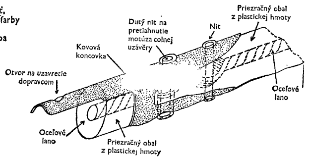
Náčrtok č. 7 Označenie kontajnerov prípustených na medzinárodné prepravy nákladov pod colnou uzáverou
